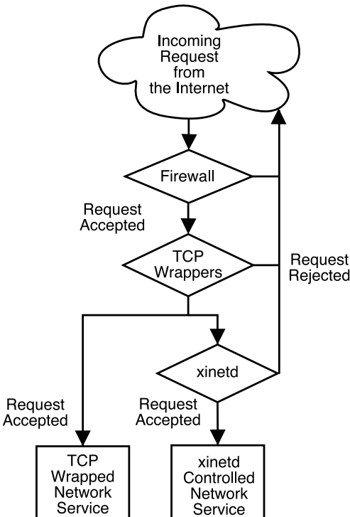
Figura 15-1. Controllo di accesso per i servizi di rete
